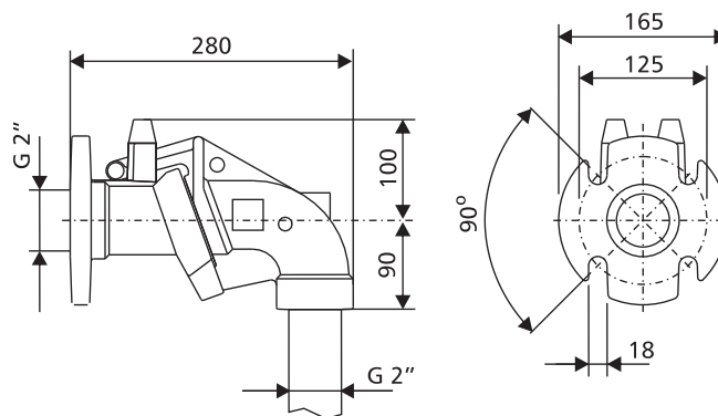
Zawiesie ZS 50
