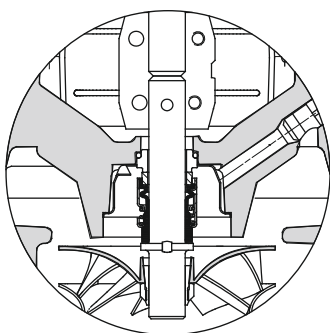
Przykładowy rysunek przekrojowy dławnicy typu BAQE
